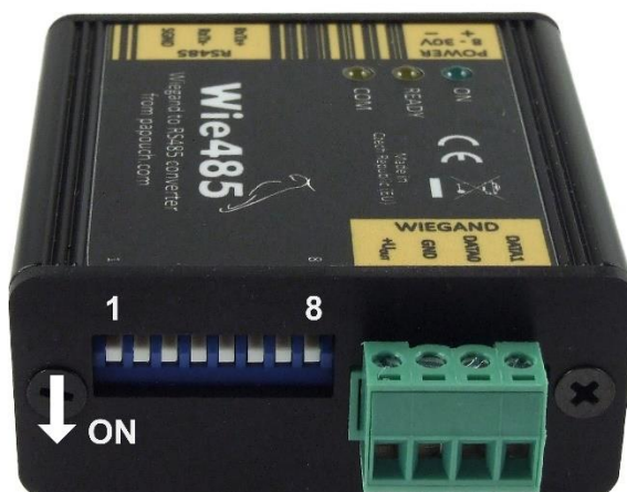
obr. 2 - umístění konfiguračních spínačů a poloha ON (sepnuto)
