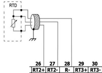
3 vodiče
