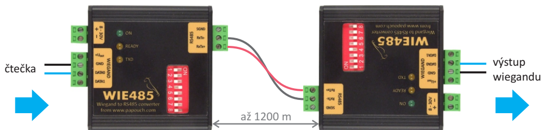
Zapojení sady prodloužení přes kroucenou dvoulinku (WiegandLong485)
