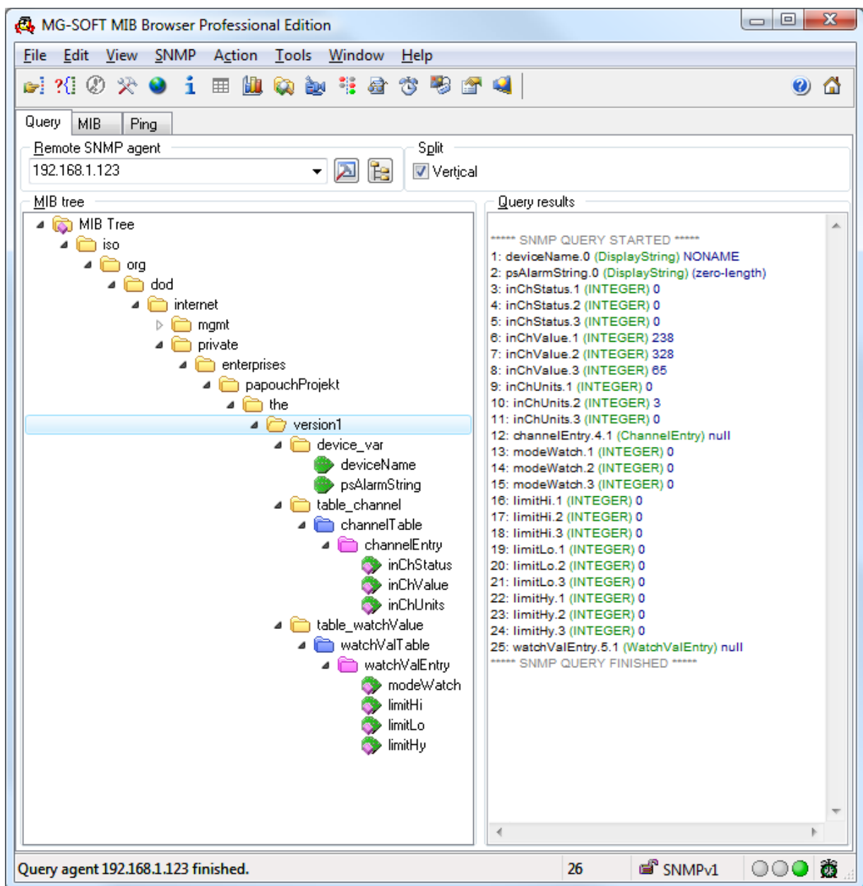
Fig. 23 – MIB tree
