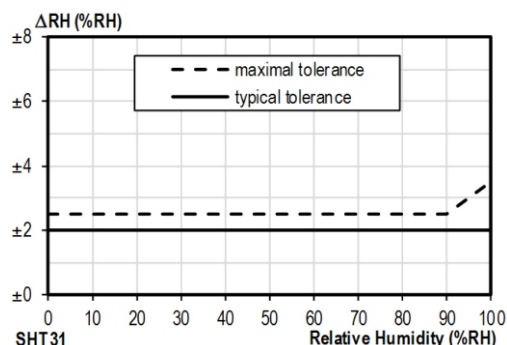
Graf 2: Přesnost měření vlhkosti
