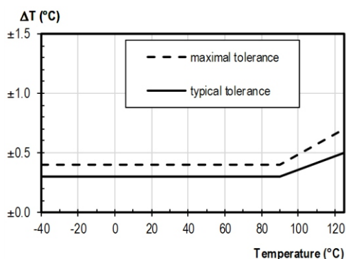
Graf 1: Přesnost měření teploty
