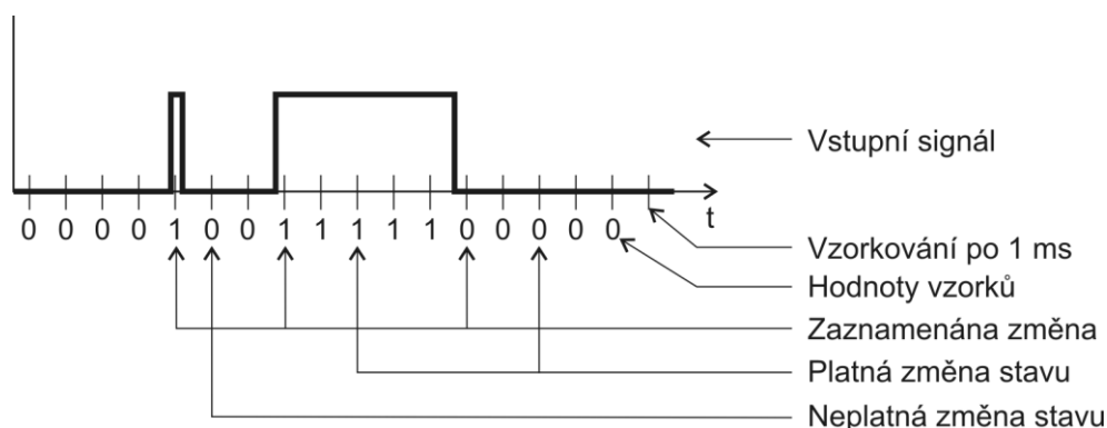
obr. 34 – princip vyhodnocování změn na vstupech
