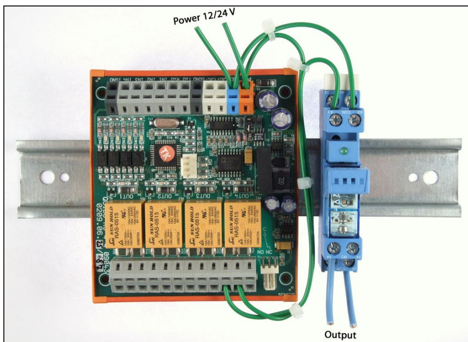
obr. 32 – Příklad zapojení Quida pro spínání 230 V AC
