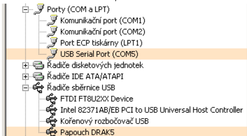
obr. 21 – správce zařízení
