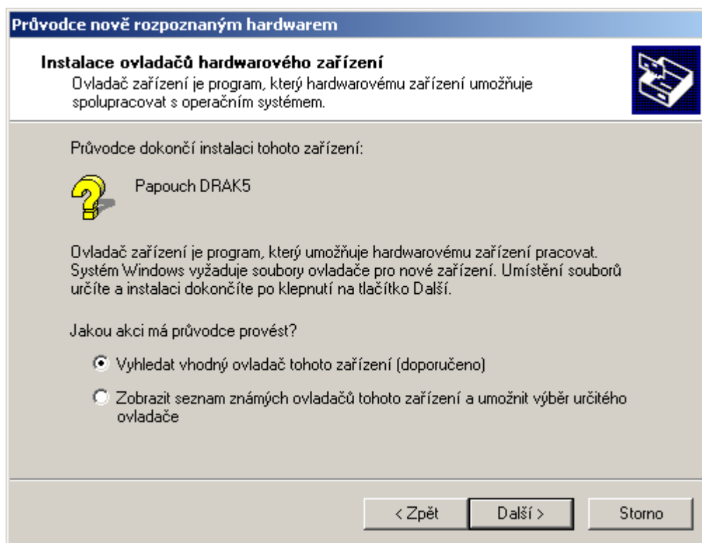
obr. 8 – Vyhledání ovladačů
