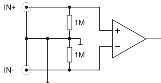
obr. 2 – náhradní zapojení měřicího vstupu
