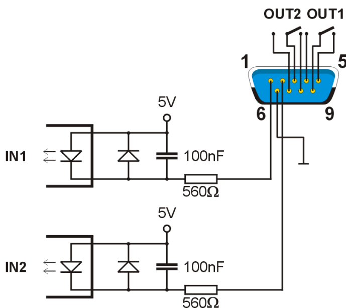
obr. 4 – zapojení digitálních vstupů a výstupů
