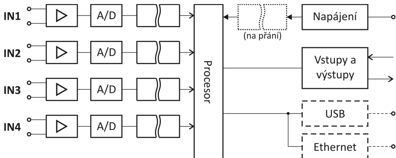
obr. 1 – blokové zapojení
