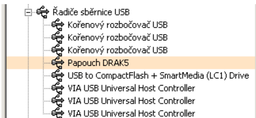
obr. 12 – správce zařízení
